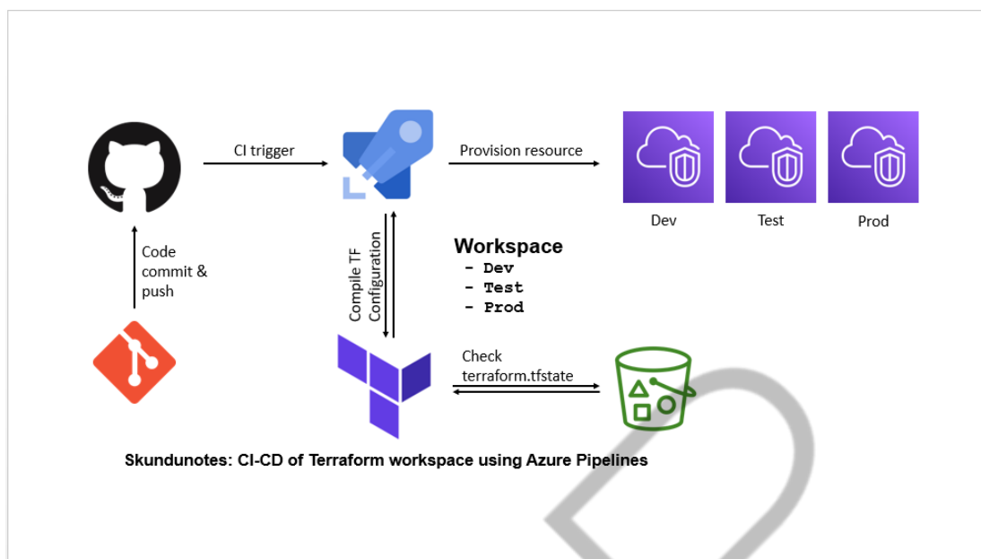
Figura 3 – Terraform State
