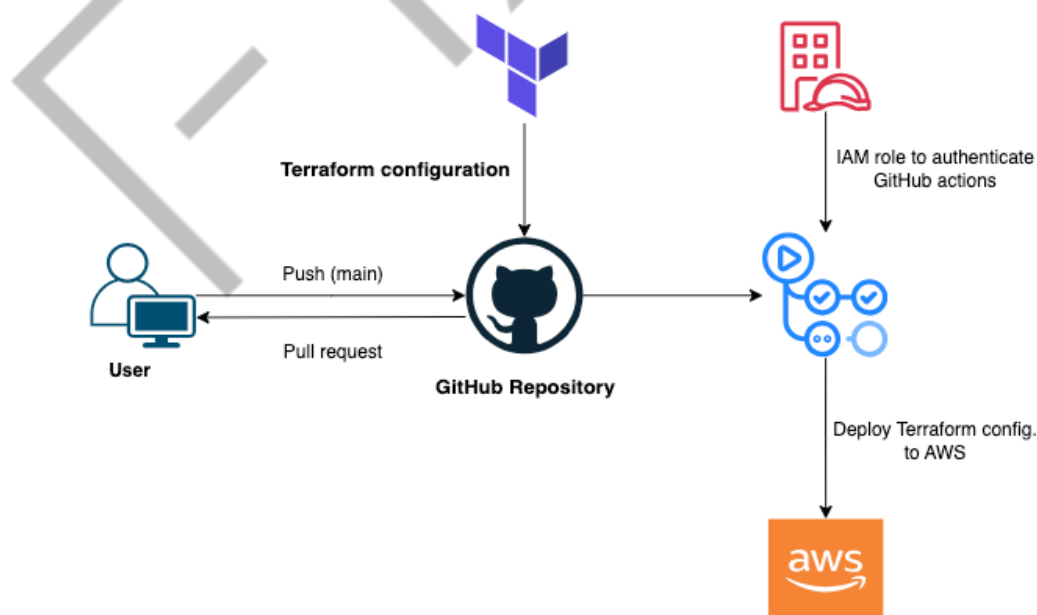
Figura 1 – CI/CD Terraform
